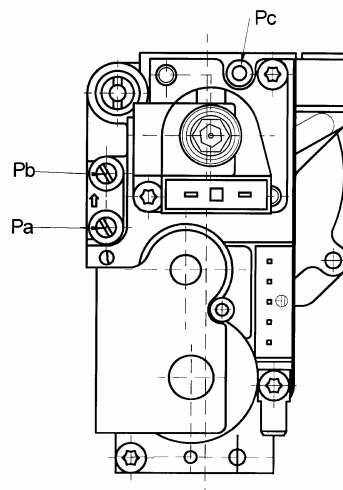
клапан Honeywell модель VK 4105 M
